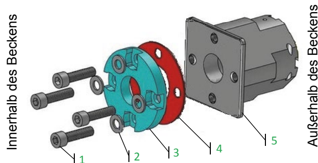
Abbildung 38 – Montage des Flansches für die Wanddurchführung
