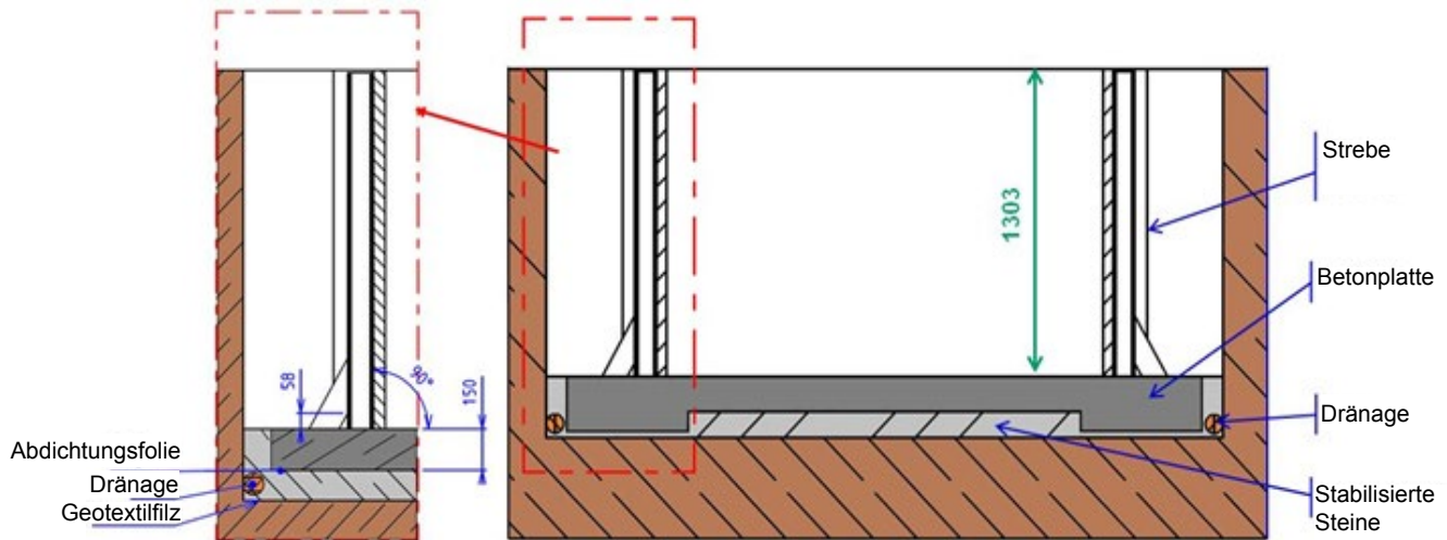
Abbildung 6 – Eigenschaften der Betonplatte
