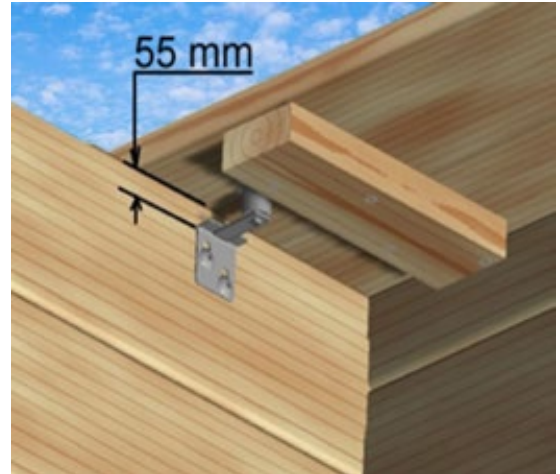
Abbildung 69 – Montage des Schließmechanismus
