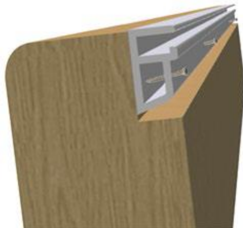
Figure 18 – Pose du rail d'accrochage
