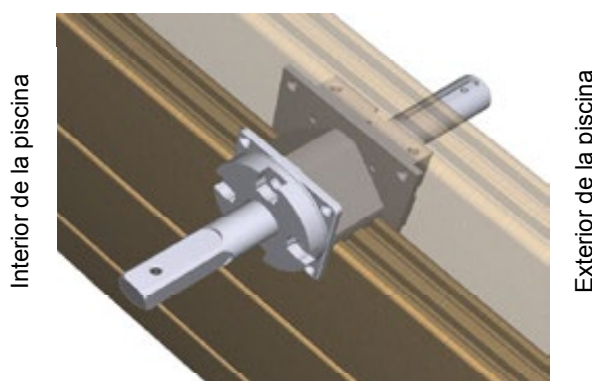
Figura 39 – Montaje del árbol de cubierta automática
