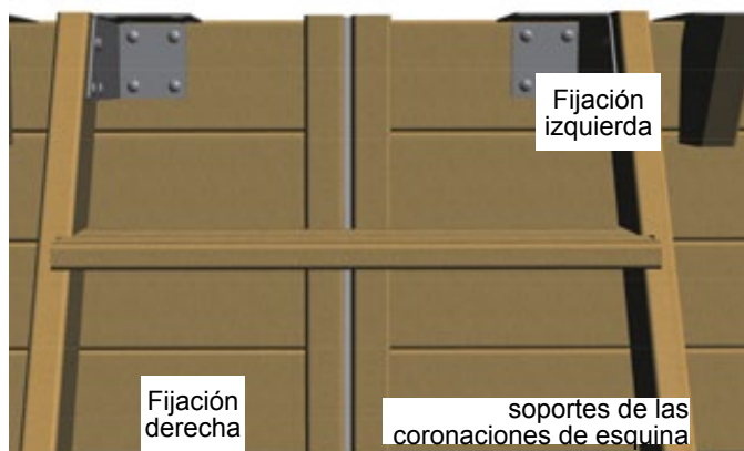
Figura 17 – Fijación de la escalera exterior sobre el vaso
