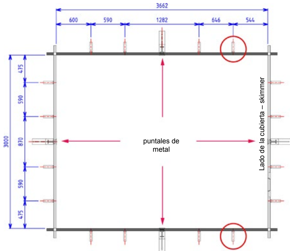
Figura 15 – Ubicación de las consolas de la coronación
