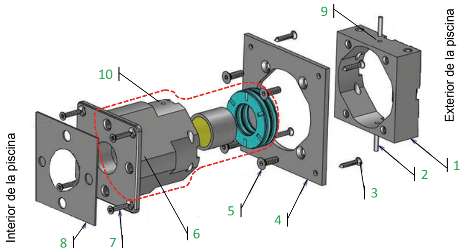
Figura 26 – Ubicación del pasamuros
