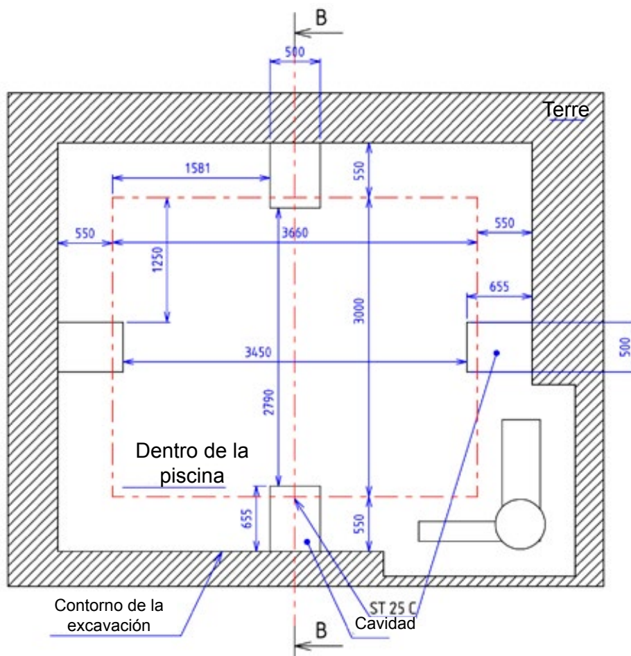
Figura 2 – Ubicaciones de cavidades para acomodar los puntales
