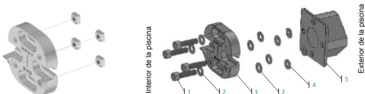
Figura 37 – Montaje de la brida porta-cojinete
