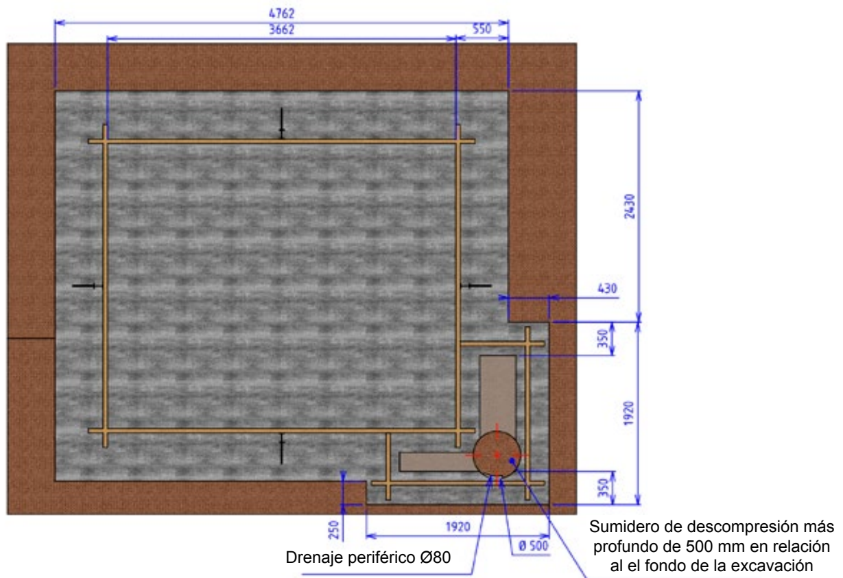
Figura 1 – Disposición del sistema de drenaje
