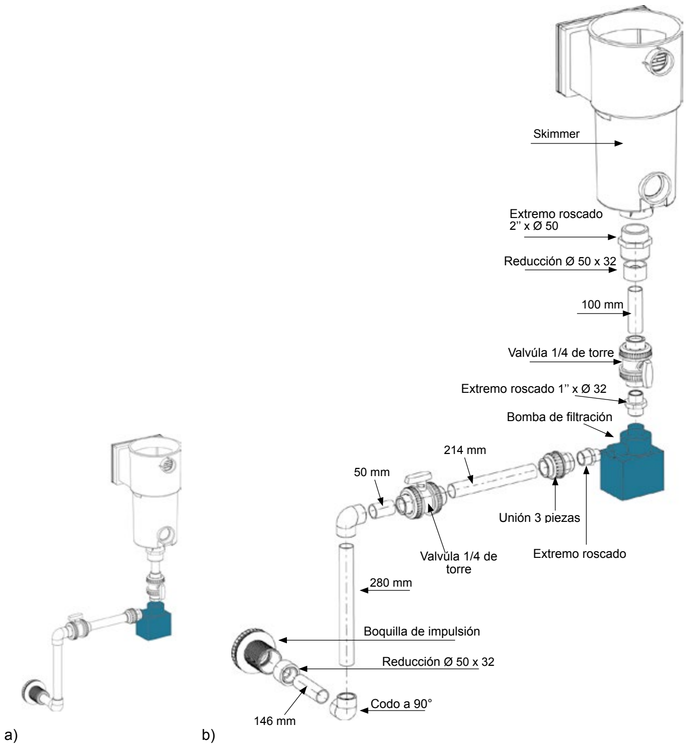
Figura 25 – a y b Tubería para la filtración
