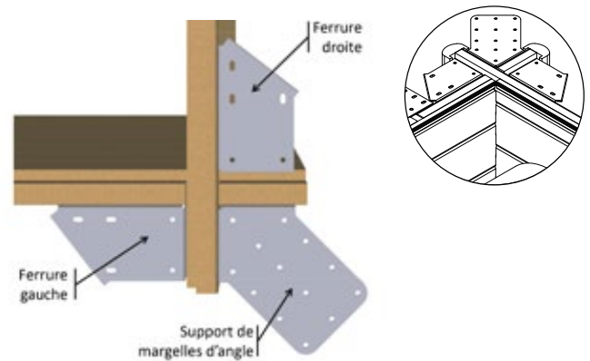
Figura 18 – Colocación de los herrajes en la parte superior de los puntales Figura 19 – Colocación de herrajes en esquinas
