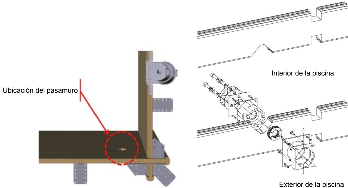
Figura 26 – Ubicación del pasamuros
