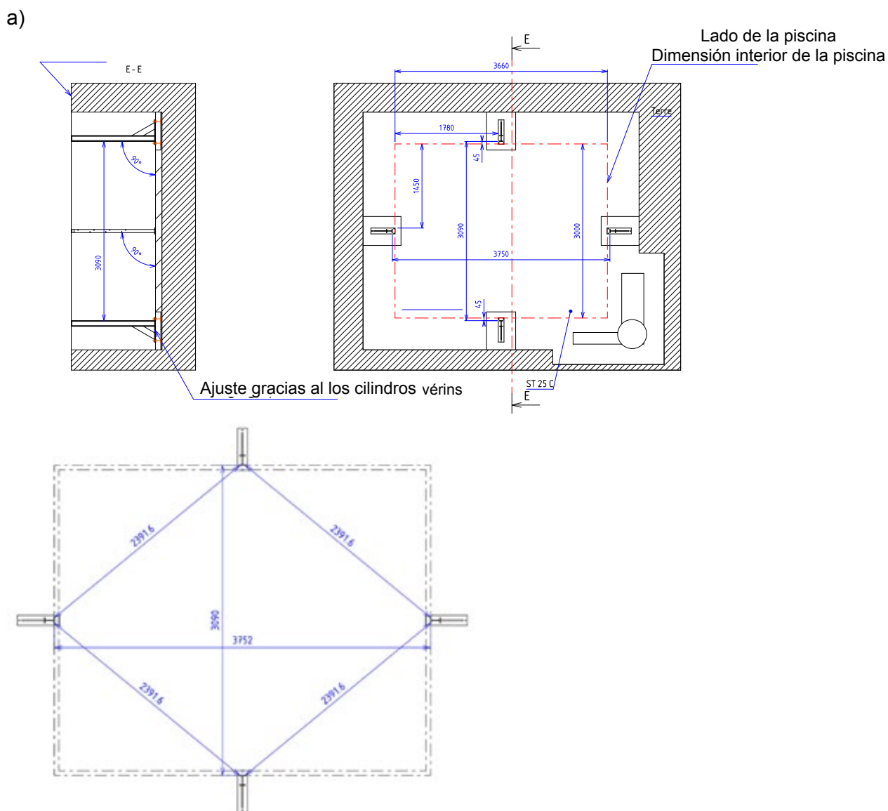
b) Figura 4 – a y b - Posicionamiento de los puntales
