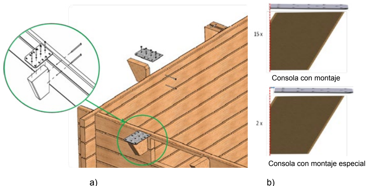
Figura 14 – a y b - Montaje de placas de metal sobre las consolas de las coronaciones
