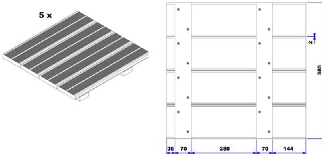
Figura 51 – Montaje de las rejillas
