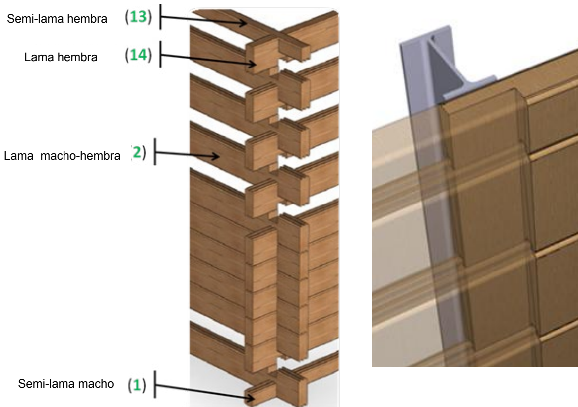
Figura 9 – Principio de ensamblaje de las láminas de madera
