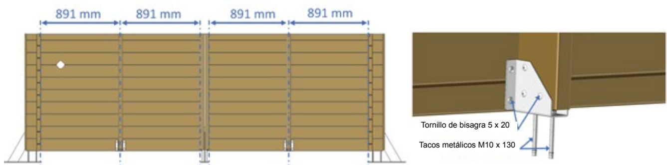
Figura 13 – Instalación de soportes y puntales de madera
