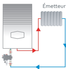
Montage sur canalisation verticale
