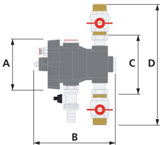
Montage sur canalisation verticale
